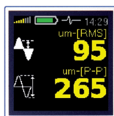
Gesamtmesswerte
