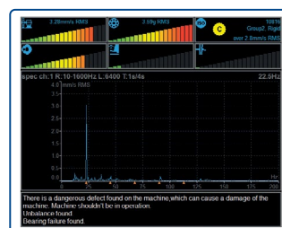
SISTEMA EXPERTO › Detección automática de fallas
