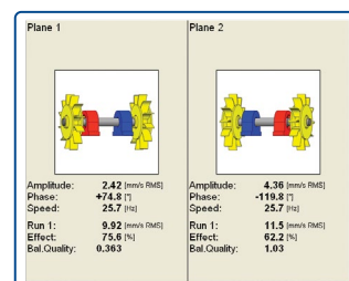
BALANCEADOR › Procedimiento de balanceo gráfico e intuitivo
