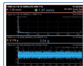
RUTA › 8000 puntos de medición › Software DDS
