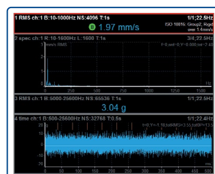
ANALIZADOR › 4 canales simultáneamente
